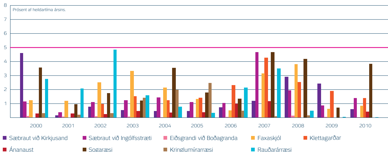
Mynd 18. Yfirfallstími fráveitu Orkuveitu Reykjavíkur
