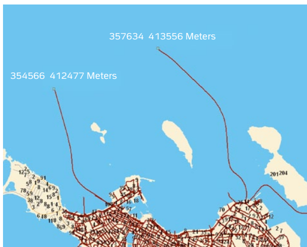
Mynd 14. Útrásir hreinsistöðvanna í Reykjavík.
