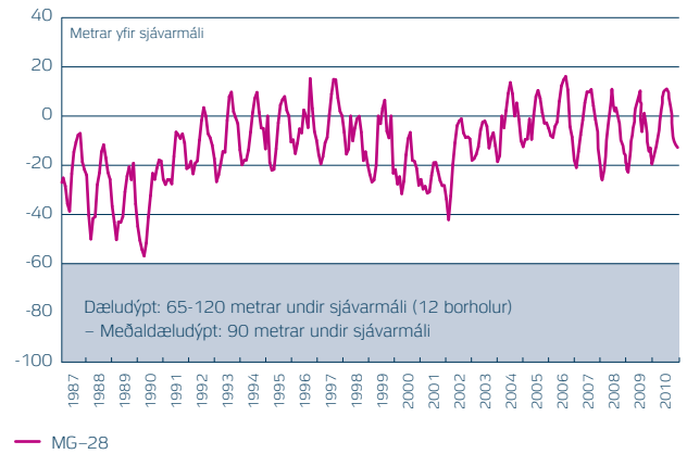
Mynd 8. Reykjahlíð, dýpt í holu MG - 28
