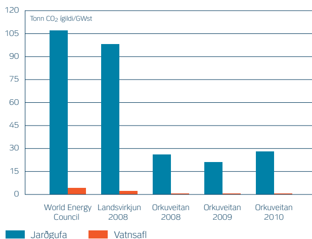
Mynd 1. Losun gróðurhúsalofttegunda á hverja framleidda GWst (CO 2 -ígildi (gr)/KWst) við rafmagnsframleiðslu með jarðvarma og vatnsafli.
