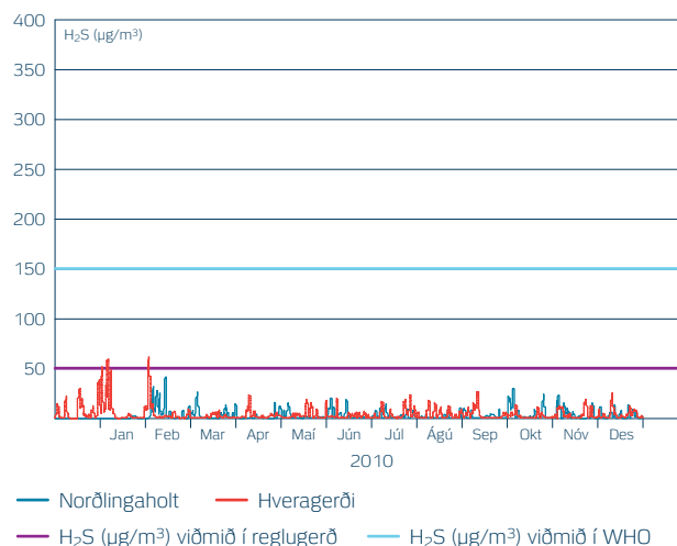
Mynd 13. Hlaupandi 24 klst. meðalstyrkur brennisteinsvetnis í Hveragerði, á Norðlingaholti og við Hellisheiðarvirkjun.
