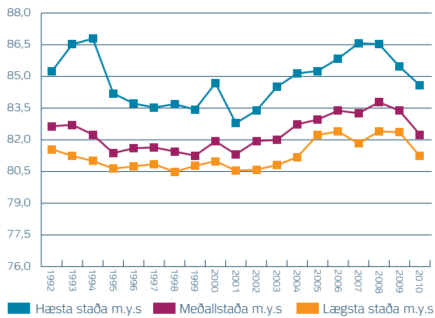
Mynd 5. Grunnvatnsstaða holu V18 á árunum 1992 til 2008. Viðmiðunarmörk eru að staðan fari aldrei undir 80 m.y.s.
