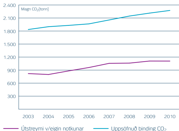
Mynd 2. Árleg binding CO 2 vegna gróðursetningar OR og útstreymi CO 2 vegna eigin notkunar (bílar, varafi og kyndistöð)
